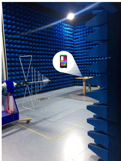
图 5-5 辐射测试图
