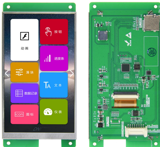
图 1-2 5.0 寸无触摸参考图
