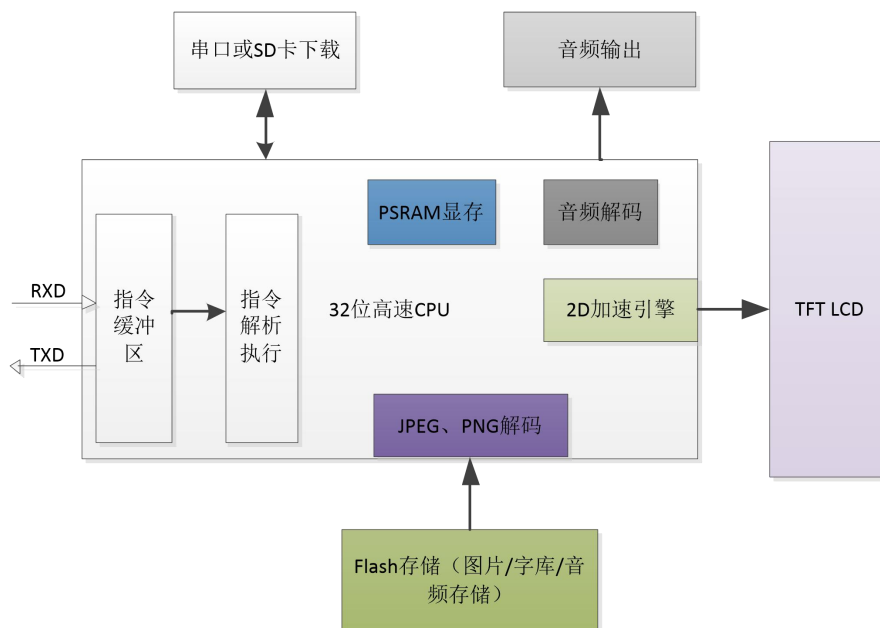
图 2-1 DN 系列串口屏内部结构图
