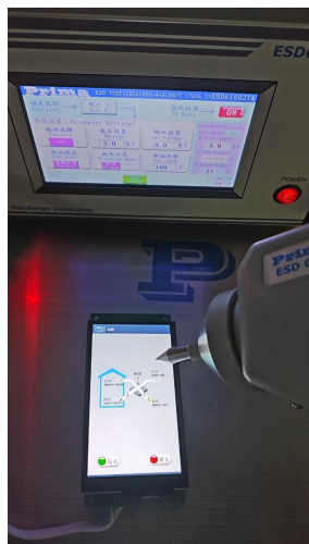
图 5-2 ESD 测试图
